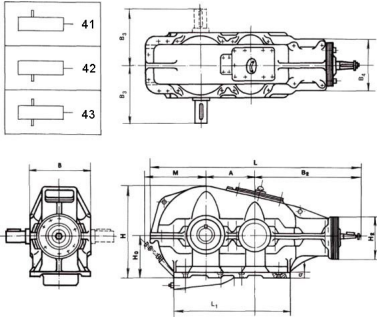
Варианты сборки по ГОСТ 20373
